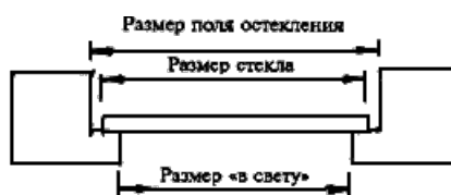
Рисунок А.1 - Определение размеров светопрозрачного заполнения
